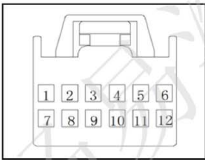
接顶灯-右后
